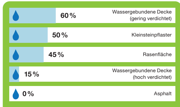
Versickerungsanteile am Niederschlag für verschiedene Belagsarten (Durchschnittswerte)
