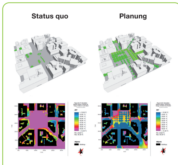
Der Simulationsvergleich von Bestandssituation und Umgestaltung zeigt, wie sich der thermische Komfort durch die Baumpflanzungen verändert. (Simulation ENVI-MET für einen Platz in der Athener Innenstadt)
