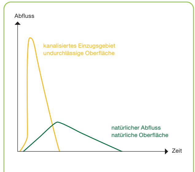
Vergleich von Abflussganglinien unterschiedlich stark befestigter und kanalisierter Gebiete. Auf natürlichen Oberflächen ist der Abfluss zeitlich gleichmäßiger verteilt, es kommt zu keinen belastenden Hochwasserspitzen.
